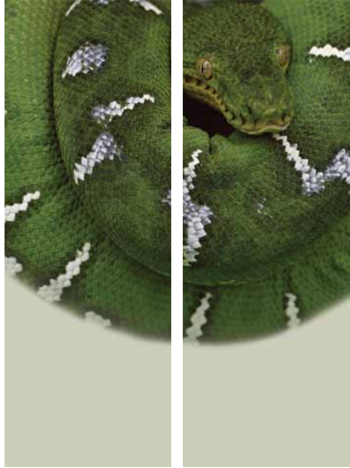
0135
